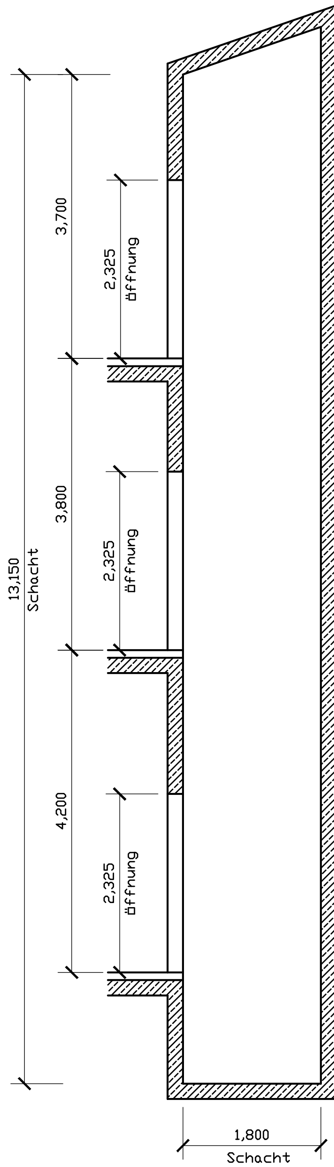
Schnitt A-A
