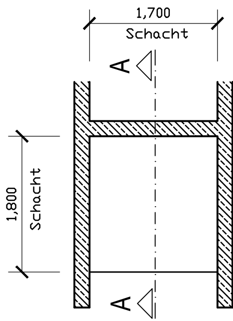
Grundriss EG, 1.OG, 2.OG
